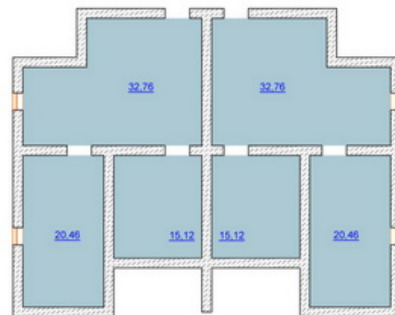
План подвала
