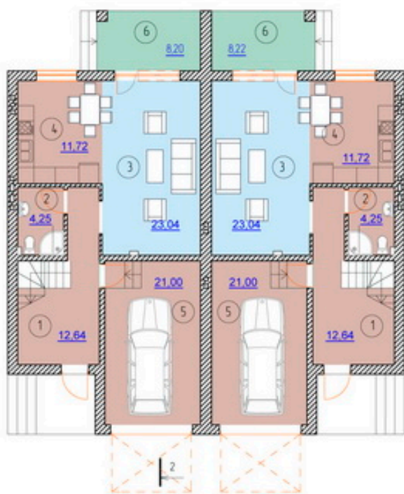
План 1 этажа
