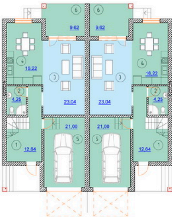
План 1 этажа
