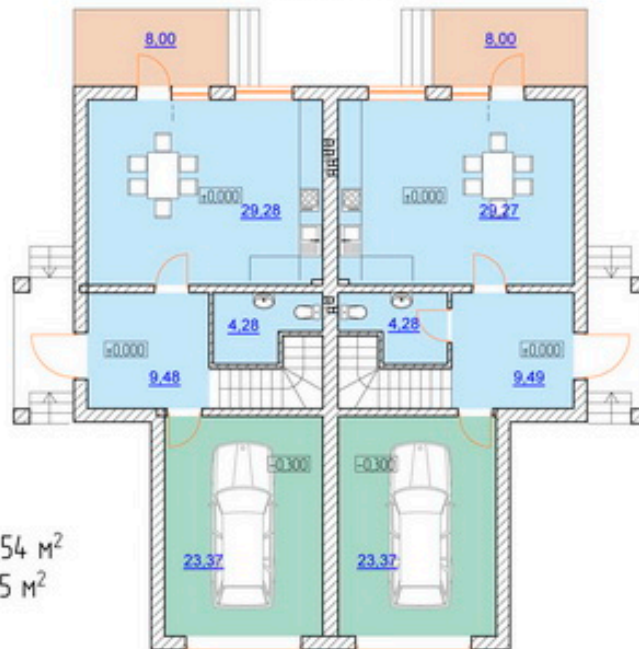
План 1 этажа
