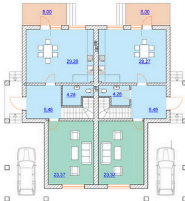
План 1 этажа
