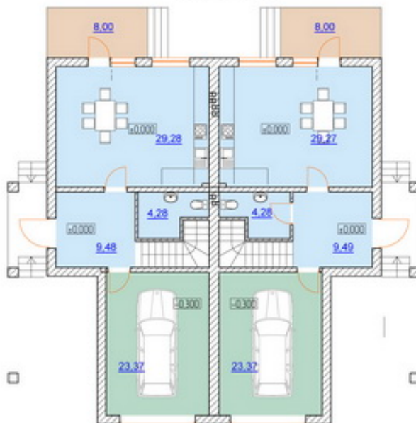
План 1 этажа
