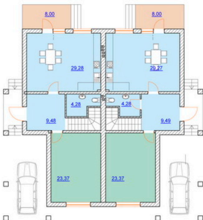
План 1 этажа
