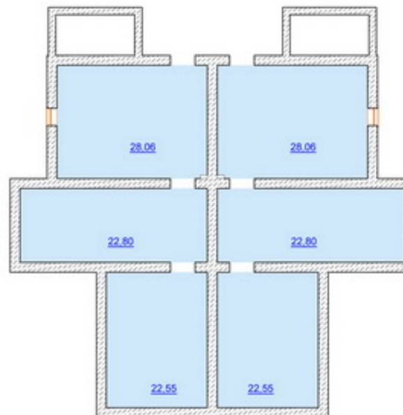
План подвала
